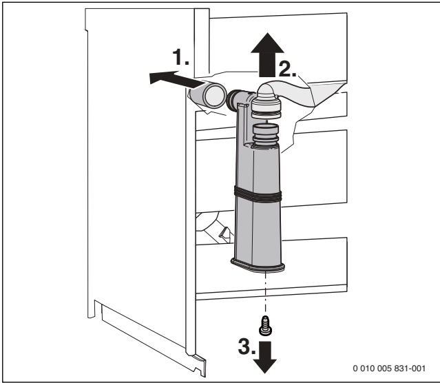
Res. 51 Yoğuşma suyu sifonunu sökme
